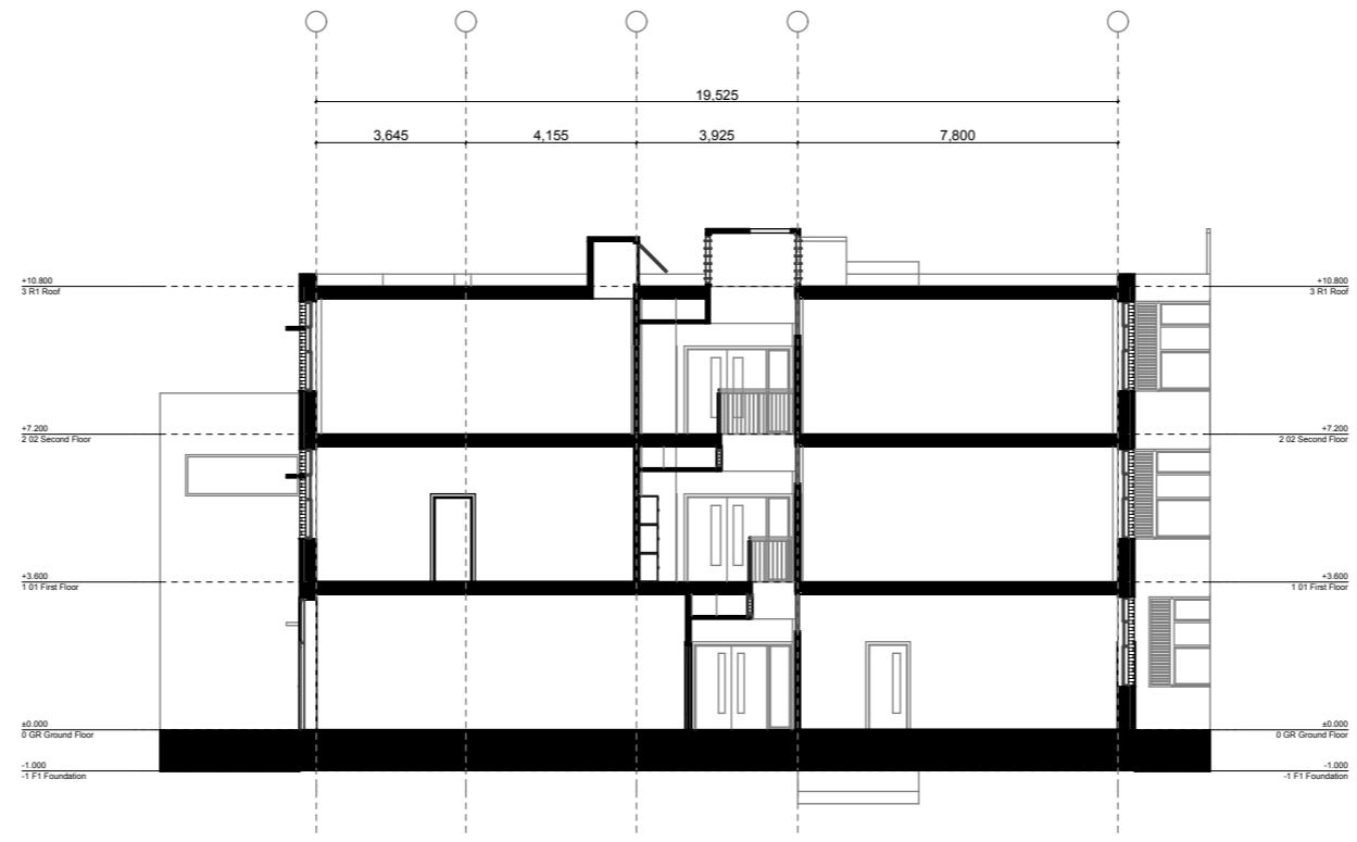
Section DD
