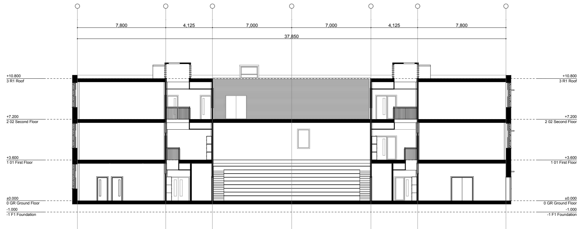
Section DD
